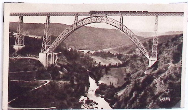
Viaduc de Garabit (Cantal) au dessus de la Bruyère, long 565m. haut 125m.
