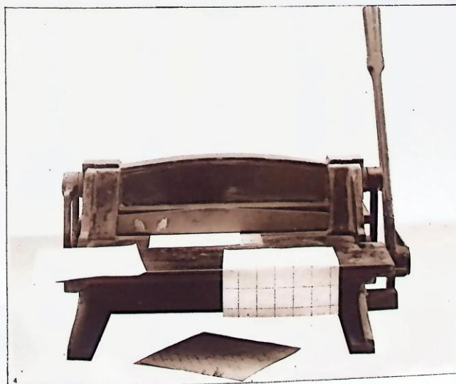
Machine à denteler les timbres.
