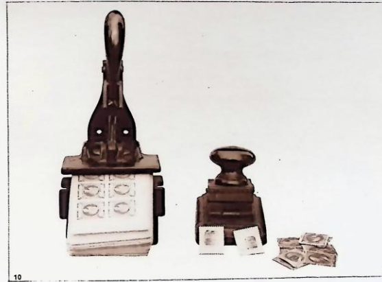
Machine à frapper la grille « Etats-Unis »
